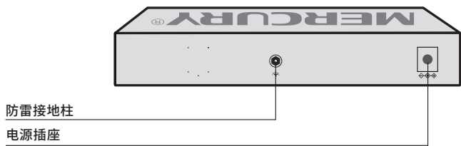
图 2-8 SE106P 后面板示意图
