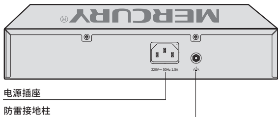
图 2-6 SE109P 后面板示意图
