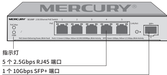
图 2-4 SE106P 前面板示意图
