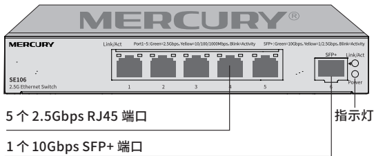
图2-2 SE106前面板示意图
